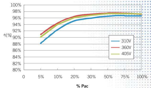
Rendementscurve voor Omniksol 2.0k-TL
